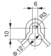
B詳細 (1:2)
