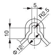
A詳細 (1:2)
