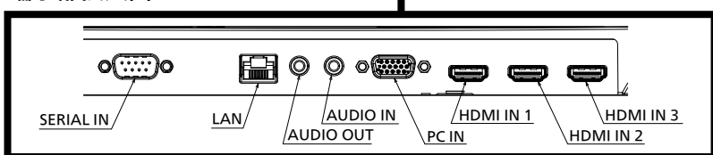
端子部拡大図 a
