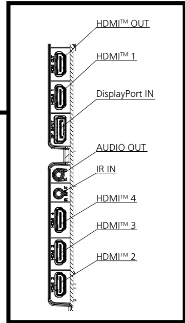
端子部拡大図b
