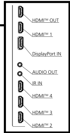
端子部拡大図 b
