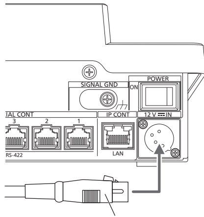
DC プラグ
