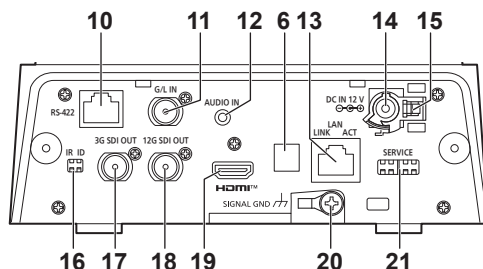
背面パネル
