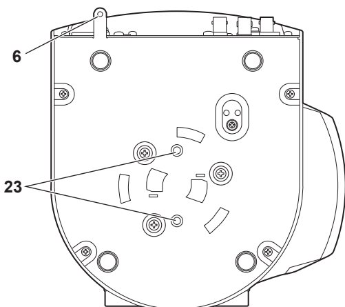
底面パネル
