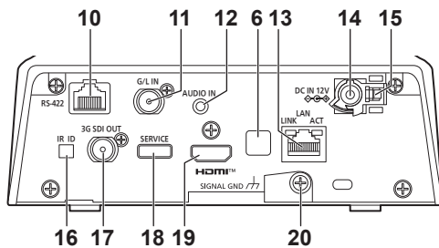
背面パネル
