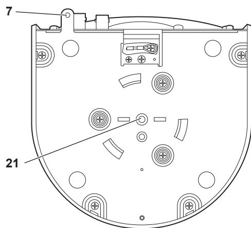
底面パネル
