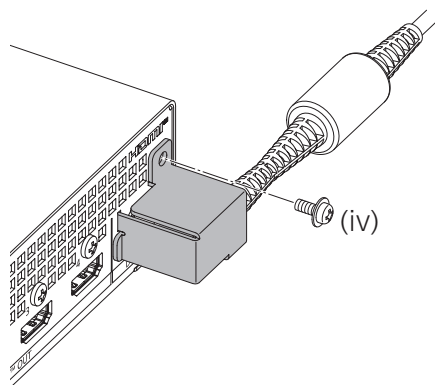
プラグを水平方向に接続した場合
