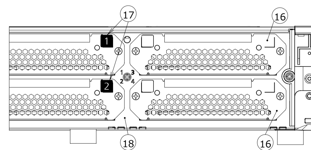
前面カバーを取り外した状態/Front cover removed WJ-NX210/2,/4
