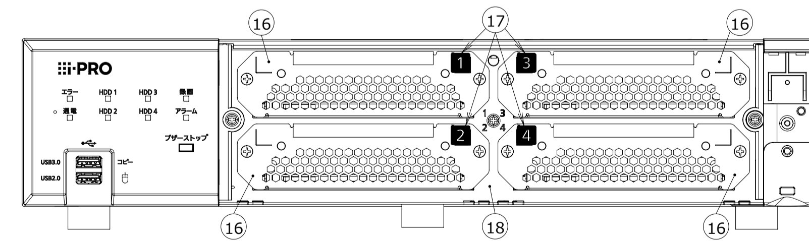
前面カバーを取り外した状態/Front cover removed WJ-NX210/8
