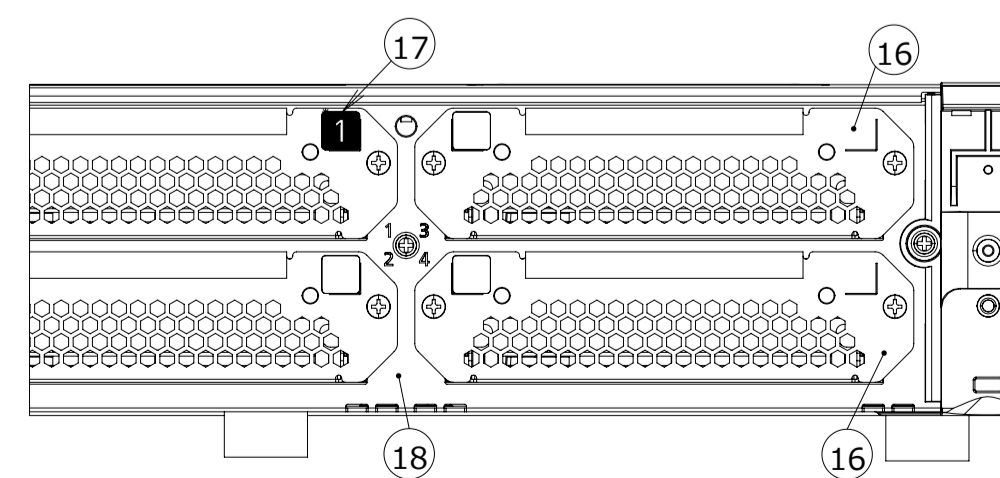
前面カバーを取り外した状態/Front cover removed WJ-NX210/1
