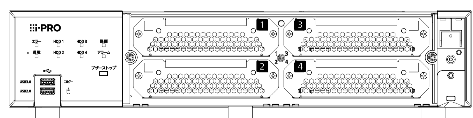
前面カバーを取り外した状態/Front cover removed WJ-NX210/8
