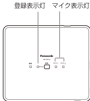
アンテナステーション (WX-SR152) 前面
