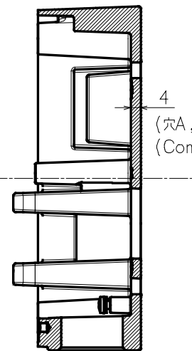
SecB-B
