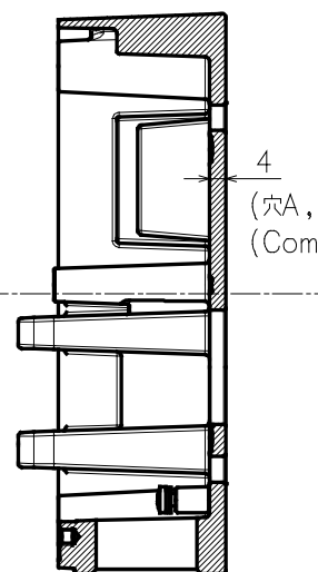
SecB-B
