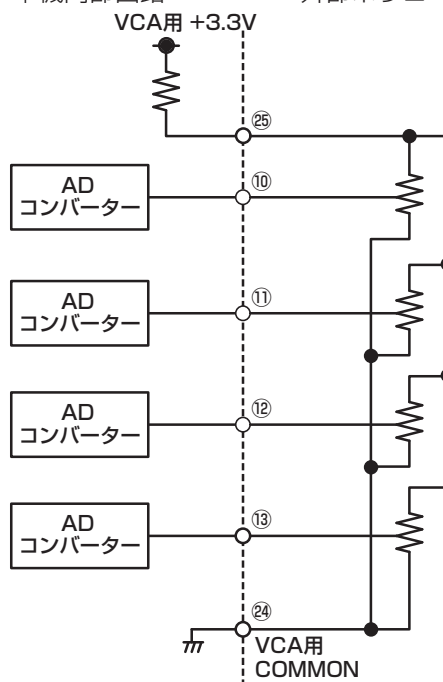
本機内部回路 外部ボリューム接続例
