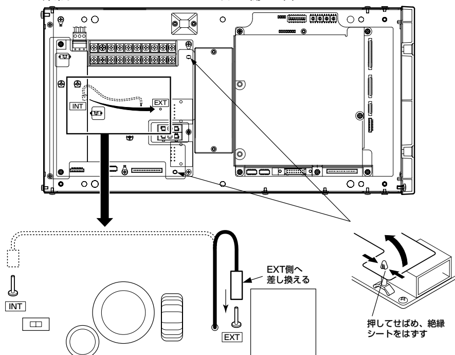
非常リモコン WR-EC500A パネルを開いた図
