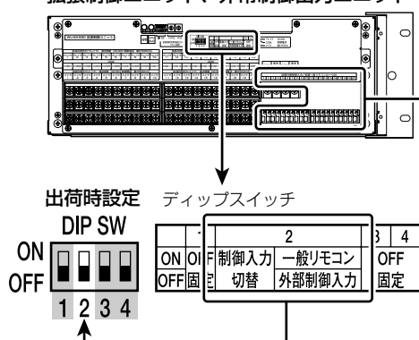
拡張制御ユニット、非常制御出力ユニット
