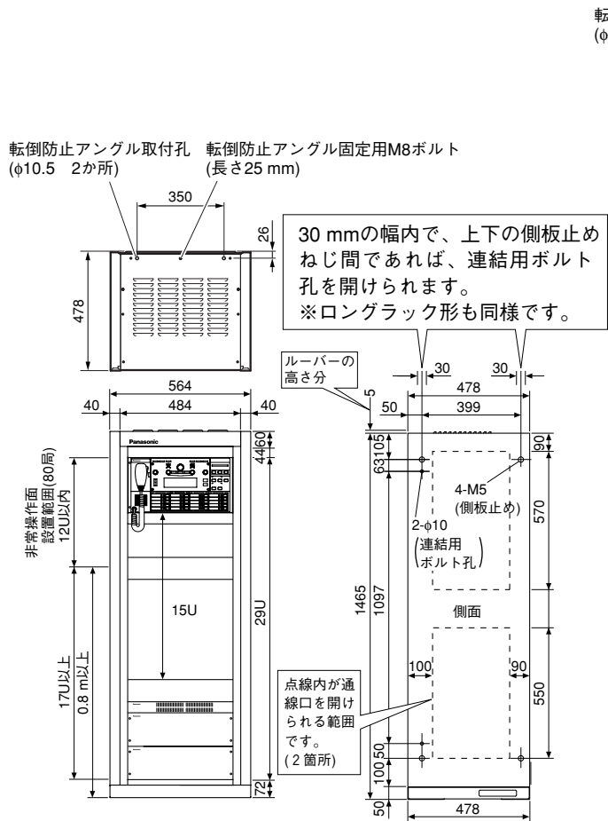
WL-8000A スタンダードラック形
