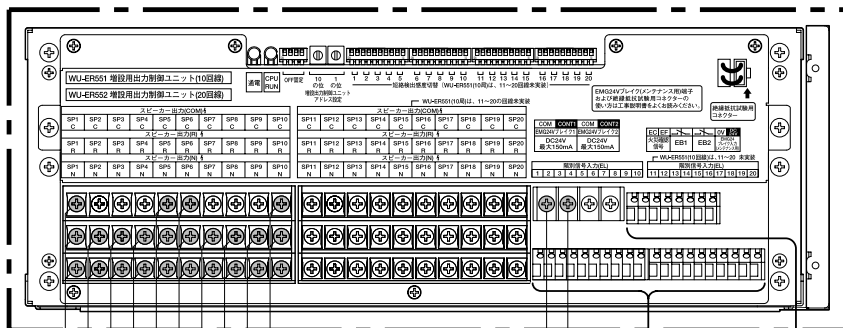
増設用出力制御ユニット WU-ER552の前面端子盤
