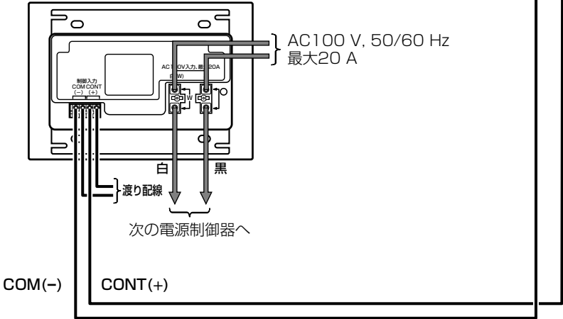
電源制御器(WU-R40B)
