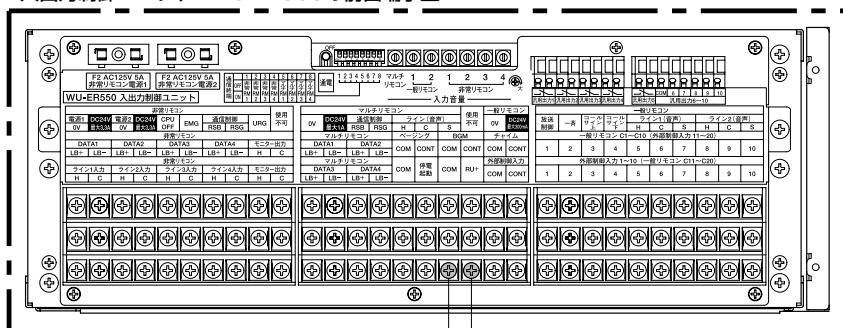
入出力制御ユニット WU-ER550の前面端子盤
