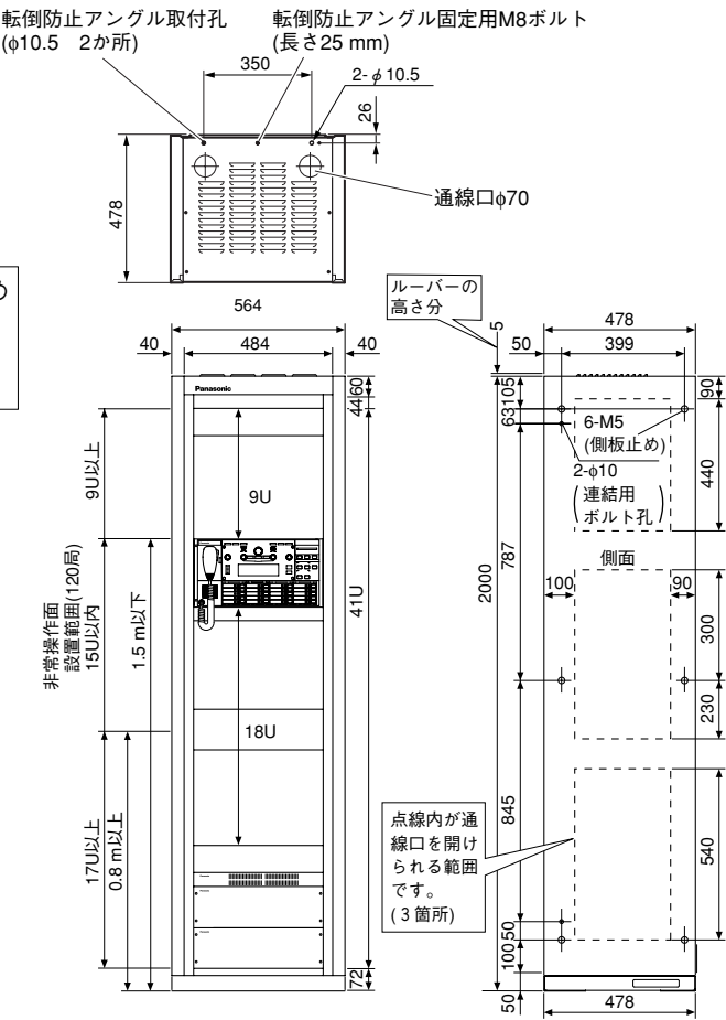
WL-8500A ロングラック形
