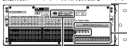
拡張制御ユニット、非常制御出力ユニット
