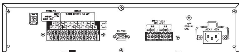
プログラムコントローラー WZ-647
