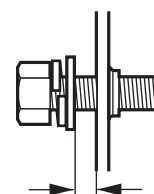
約5 mmのすき間を空けて仮止め
