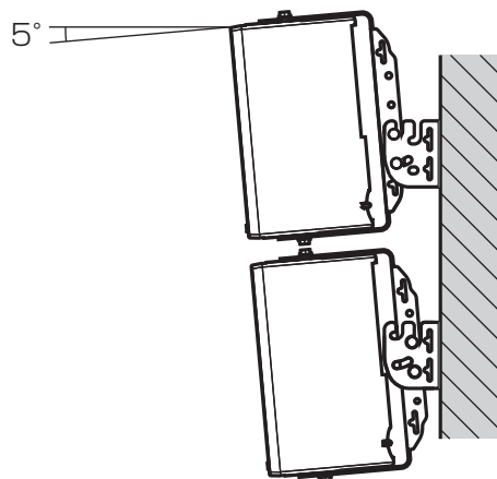
取付状態
