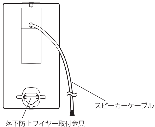
後面 (スピーカー取付金具を 外した状態)
