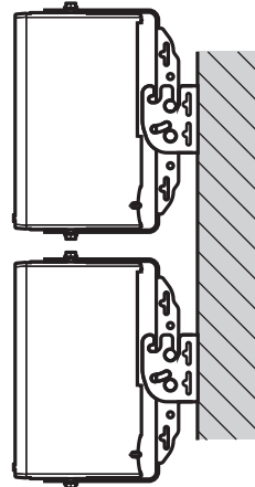
取付状態
