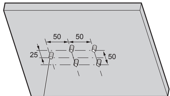
落下防止ワイヤーの 取付プレート用アンカー位置 ※アンカー位置は、固定金具 の取り付けの向きによって 異なります。（15ページ）
