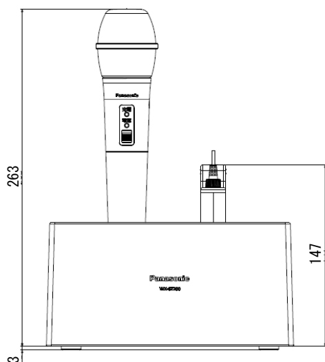
WX-ST200、WX-ST400 挿入状態
