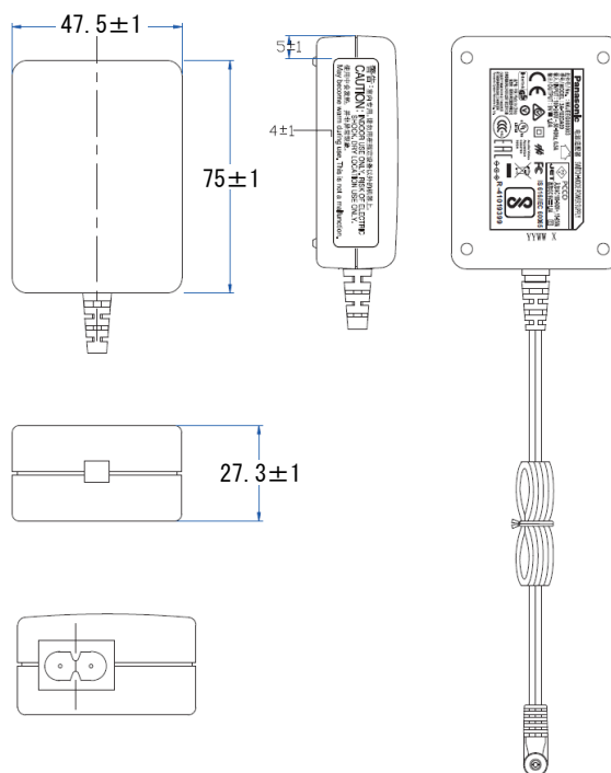
AC アダプター
