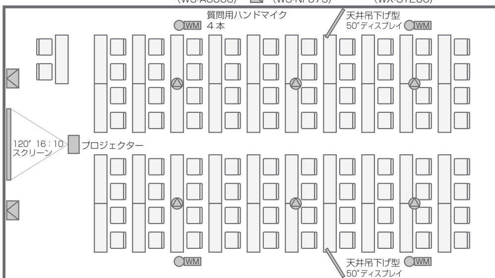
横 10 m × 奥行 18 m = 180 m 2 △ : 天井 SP (WS-AC066) ▽ : メイン SP (WS-NF075) ● WM : ハンドマイク (WX-ST200)
