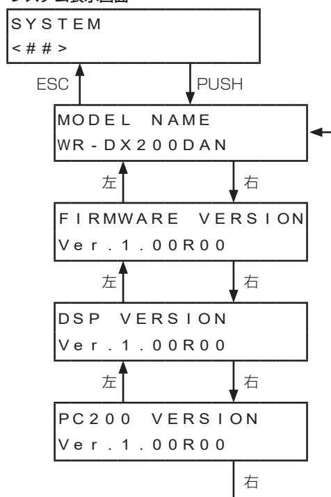
システム表示画面
