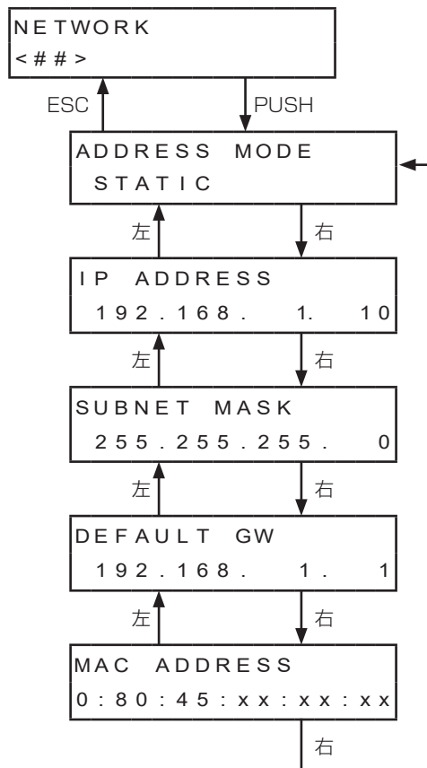
ネットワーク設定表示画面
