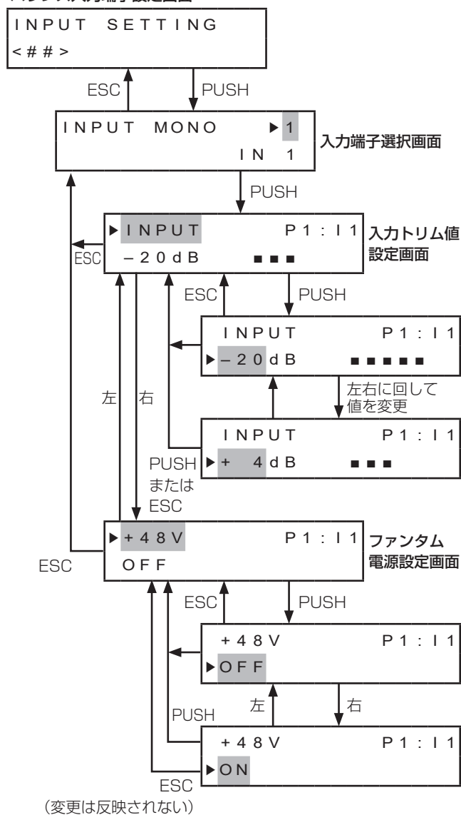
バランス入力端子設定画面
