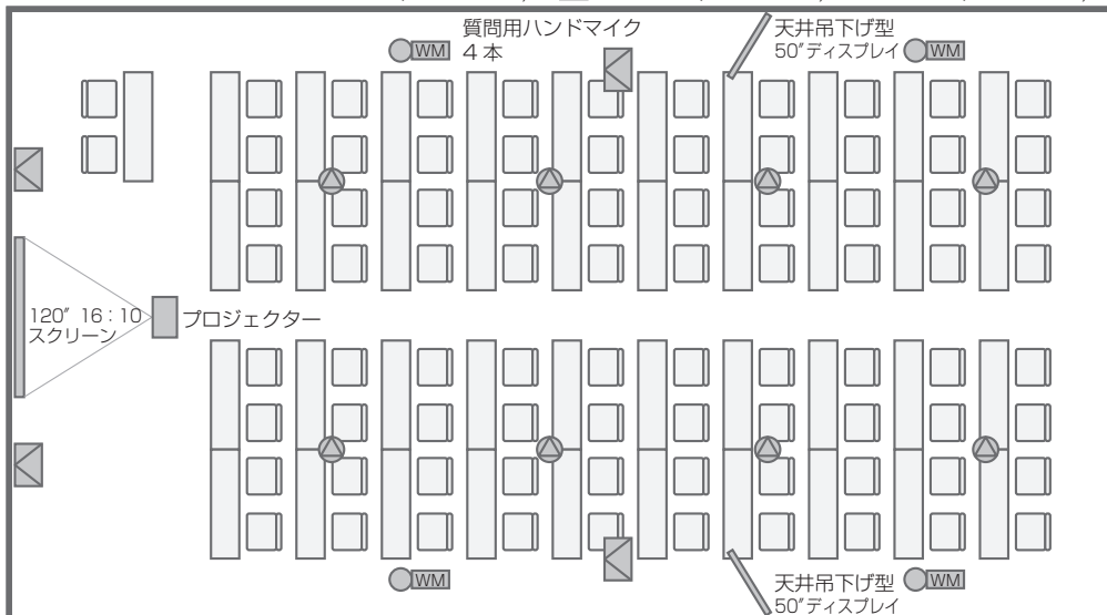
横 10 m × 奥行 18 m = 180 m 2 ● : 天井 SP (WS-AC066) ◻ : メイン SP (WS-NF075) サブ SP (WS-NF075) ● WM : ハンドマイク (WX-ST200)
