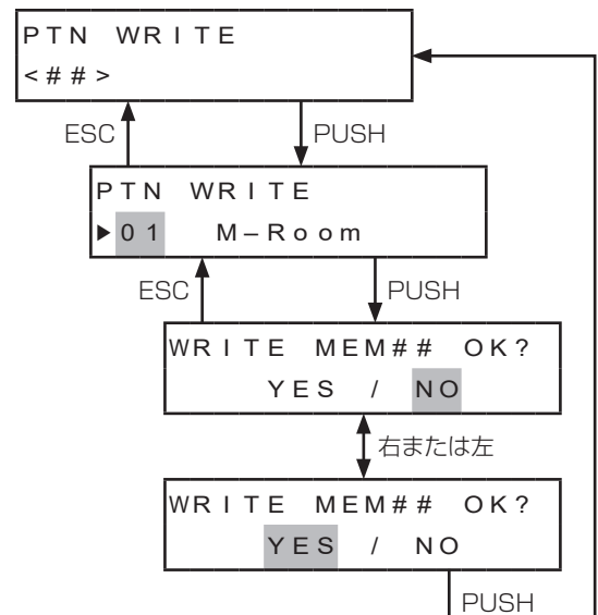
パターンメモリ書き込み画面
