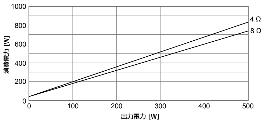
電力特性（全チャンネル出力合計）4/8 \Omega
