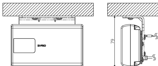
WV-QHS500-WとWV-QWL505 (金具A) の組み合わせ例
