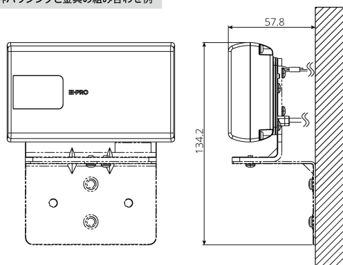
WV-QHS500-WとWV-QWL505 (金具A+金具B) の組み合わせ例
