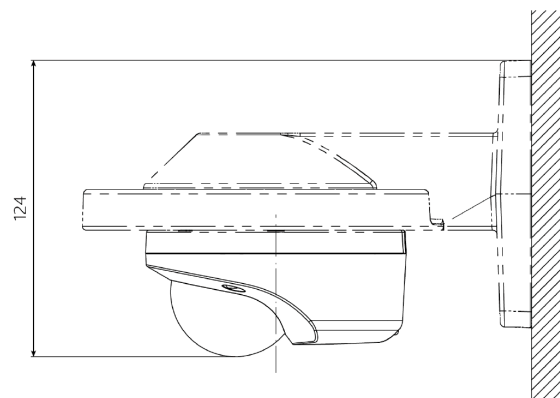
WV-QWL500-** 組み合わせ例
