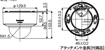
アタッチメント金具 [付属品]
