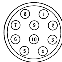
10ピンコネクタ(メス)
