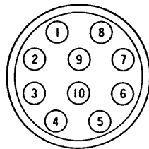
10ピンコネクタ(オス)
