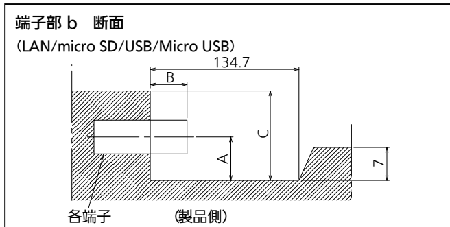
端子部 b 42AF1 側面端子
