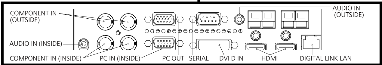
端子部拡大図 a
