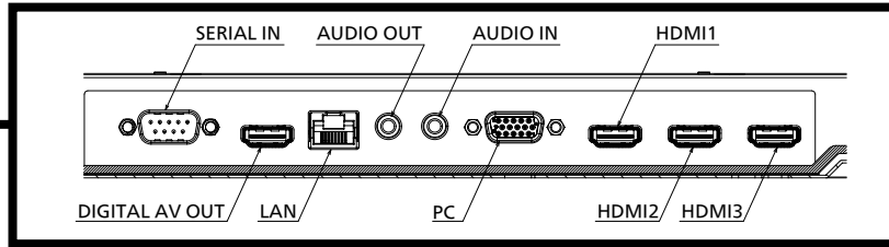
端子部拡大図 a
