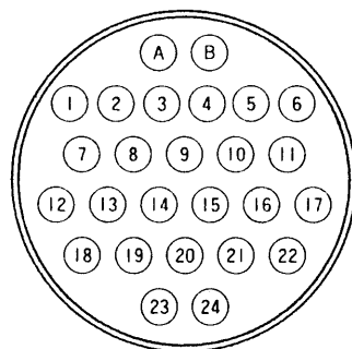
26ピンコネクタ(オス)
