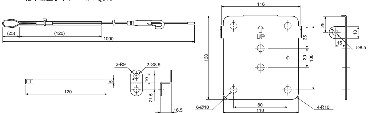
落下防止ワイヤー WV-Q140
