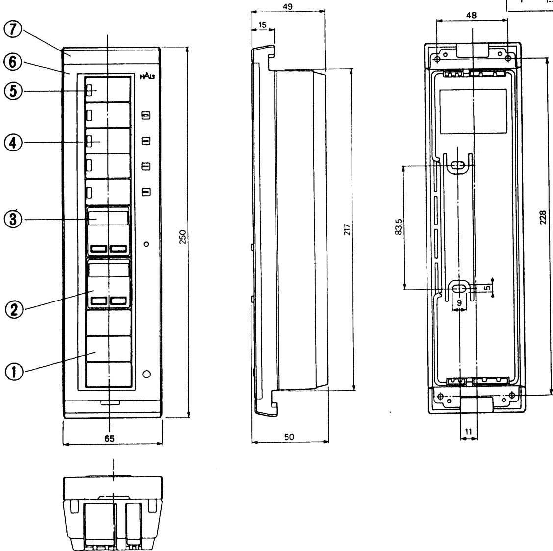
壁穴あけ寸法(尺度不適用)
