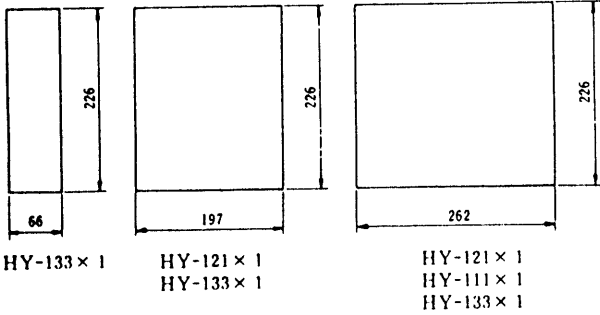
壁穴あけ寸法(尺度不適用)
