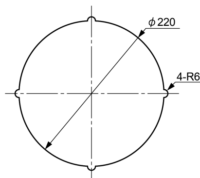
●天井加工穴寸法図
