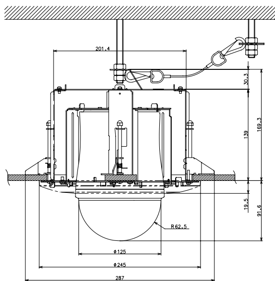
●天井加工穴寸法図
