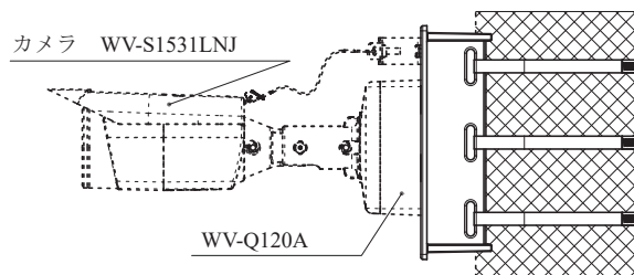
四角型のカメラ取付台を持ったアナログカメラまたは ネットワークカメラをWV-Q120A (カメラ取付金具) を使って取り付ける場合
