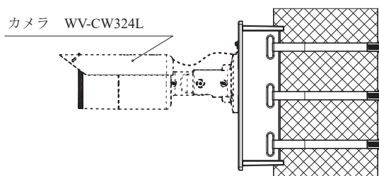
丸型のカメラ取付台を持った アナログカメラを取り付ける場合
