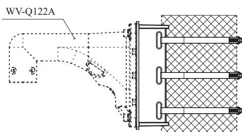
WV-Q122A (カメラ壁取付金具) を使っ てカメラを取り付ける場合
