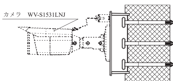
四角型のカメラ取付台を持ったアナログカメラ またはネットワークカメラを直接取り付ける場合
