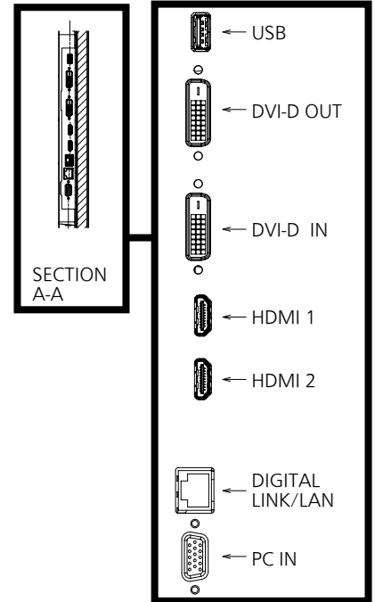
端子部拡大図a
