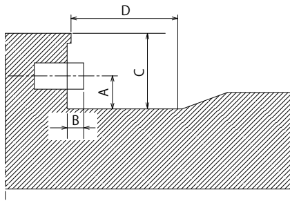
端子部 a 断面 (USB/DVI-D OUT/DVI-D IN/HDMI 1,2/DIGITAL LINK LAN/PC IN)
