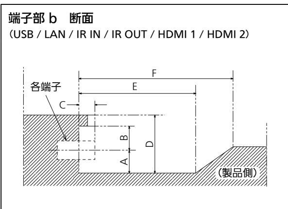
端子部 b 50EQ1J 側面端子
