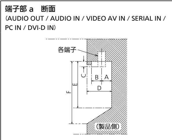
端子部 a 50EQ1J 下部端子
