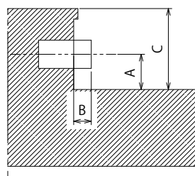
端子部 a 断面 (USB/DVI-D OUT/DVI-D IN/HDMI 1,2/DIGITAL LINK LAN/PC IN)
