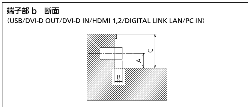
端子部 b 70SF2HJ 下部端子
