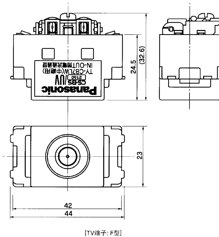
[TV端子: F型]
