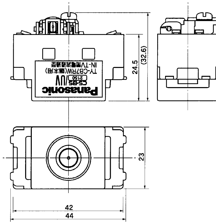
[TV端子: F型]
