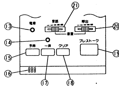
操作部詳細
