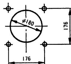
取付孔図
