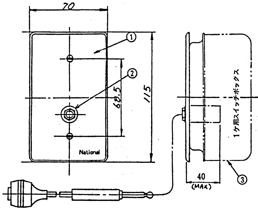
適合呼出にぎり押釦(VH-804J)
