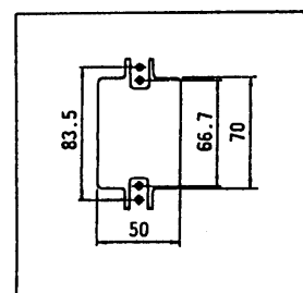
取り付け穴寸法 1/5
