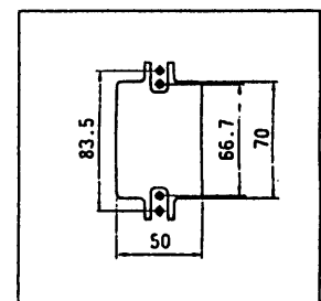
取り付け穴寸法 1/6
