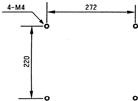
取付穴寸法
