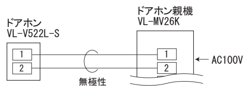
《配線図》
