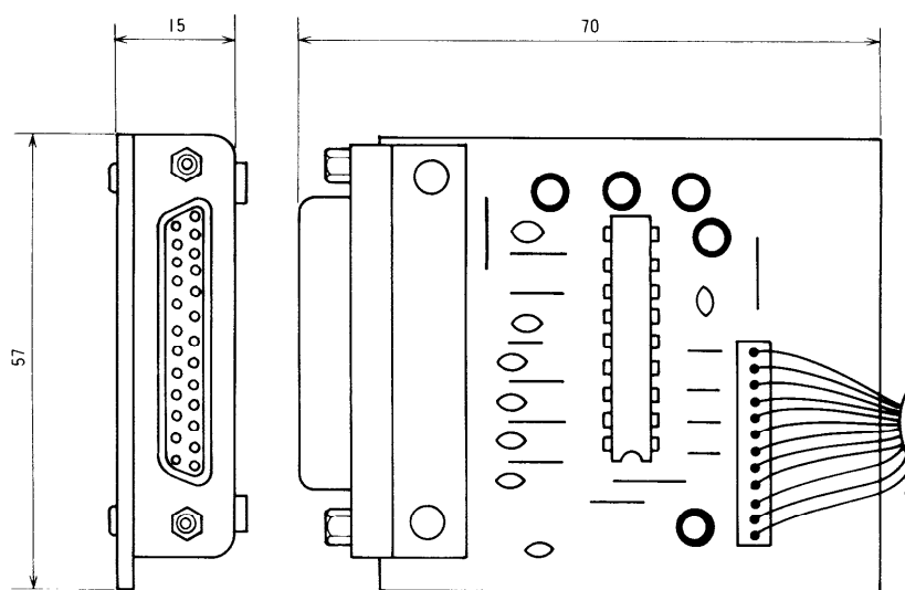
RS-232Cボード
