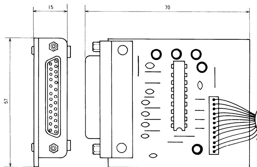
RS-232Cボード
